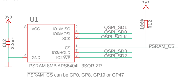
PSRAM
